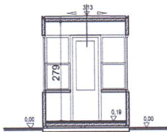
PRESJEK
